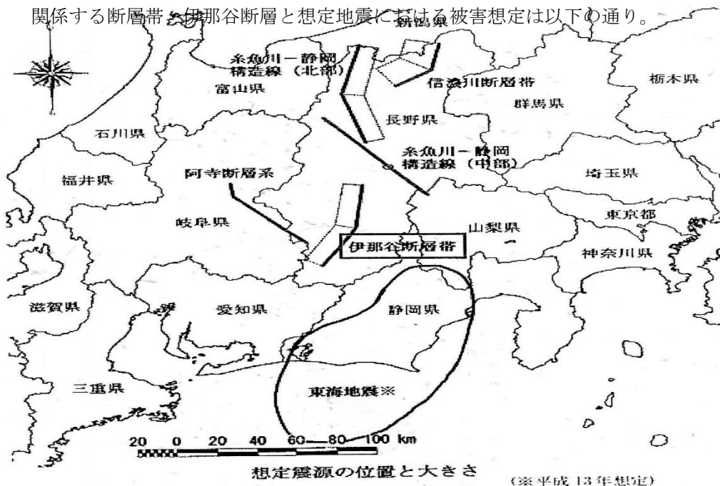
想定地震の震源位置と大きさ（長野県地域防災計画より抜粋）
