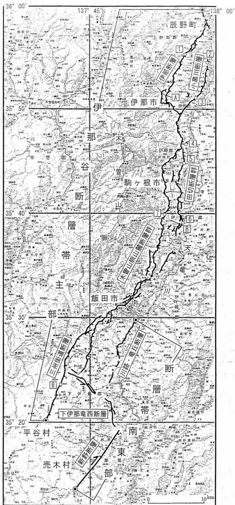
伊那谷断層帯の位置と主な調査地点
