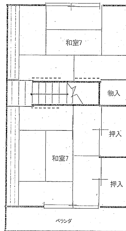
2階平面図
