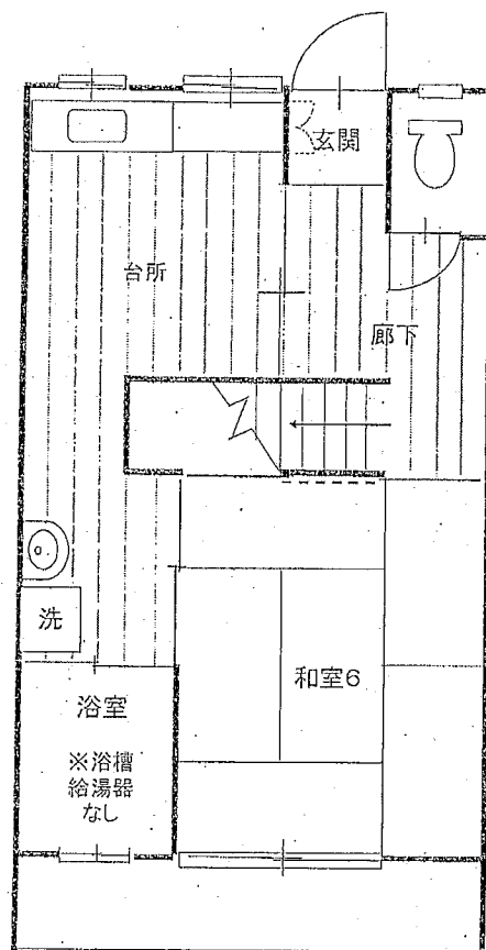
1階平面図
