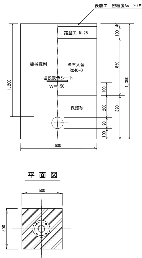
掘削断面図（道路部）
