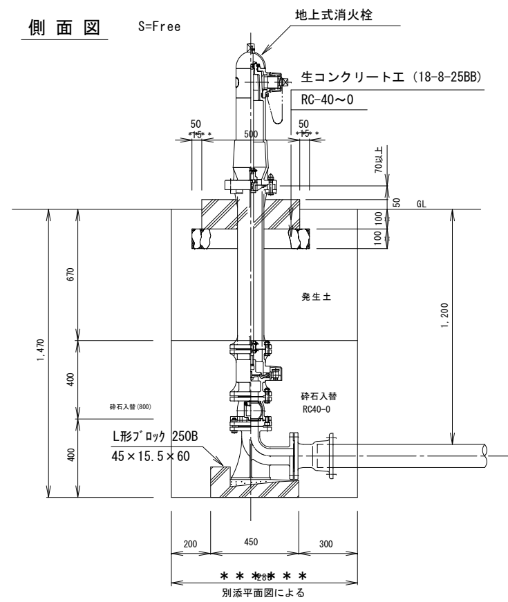
参考：掘削断面図（消火栓部）
