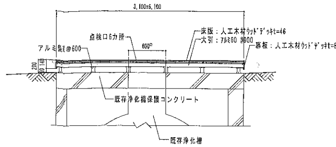
緑地内ウッドデッキ詳細図 S=1/30
