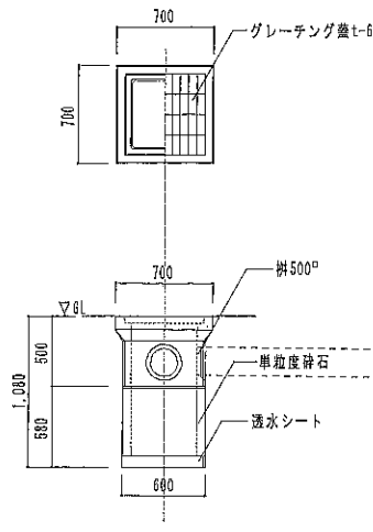
柵C詳細図 S=1/30
