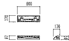
車止め詳細図 S=1/30
