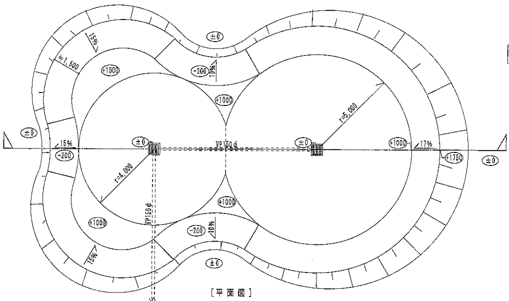
パントラックコース詳細図 S=1/100
