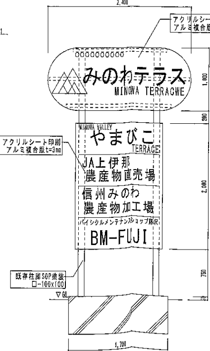
既存看板A詳細図 S=1/30
