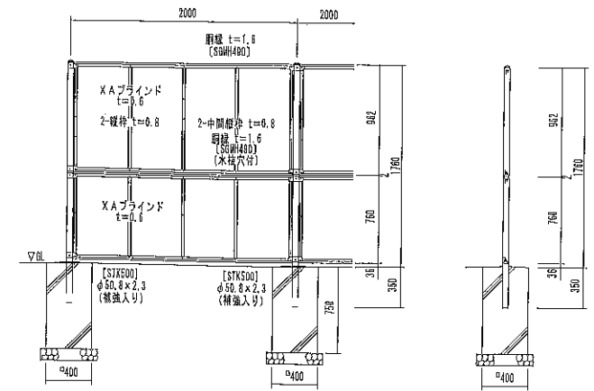
フェンス詳細図A S=1/30
