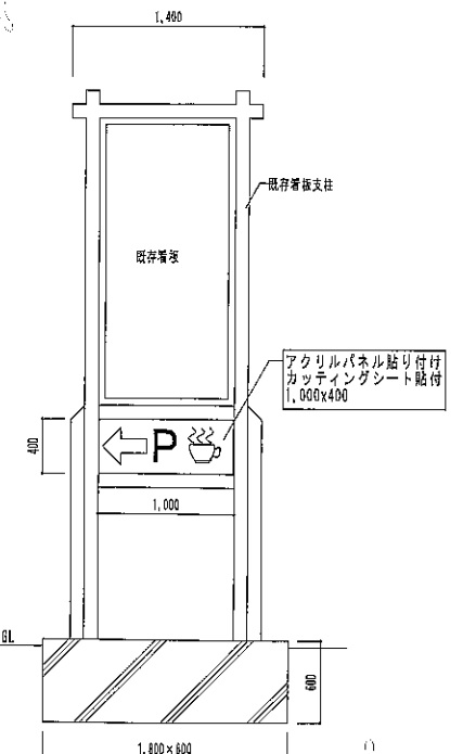
既存看板C詳細図 S=1/30
