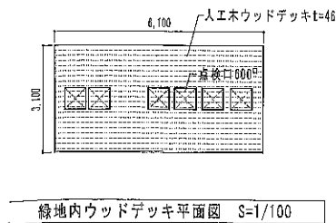
緑地内ウッドデッキ平面図 S=1/100
