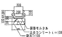
ベンチフリーム300詳細図 S=1/30
