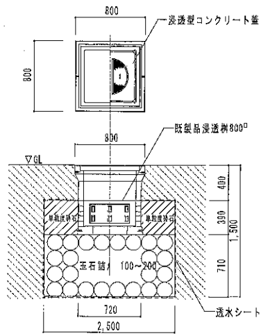
浸透性詳細図 S=1/30
