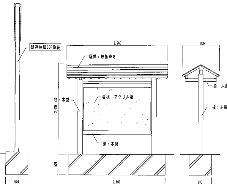
既存看板B詳細図 S=1/30
