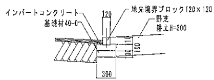
地先境界ブロック詳細図 S=1/30
