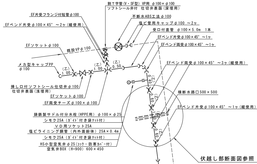
配管詳細図 S=FREE
