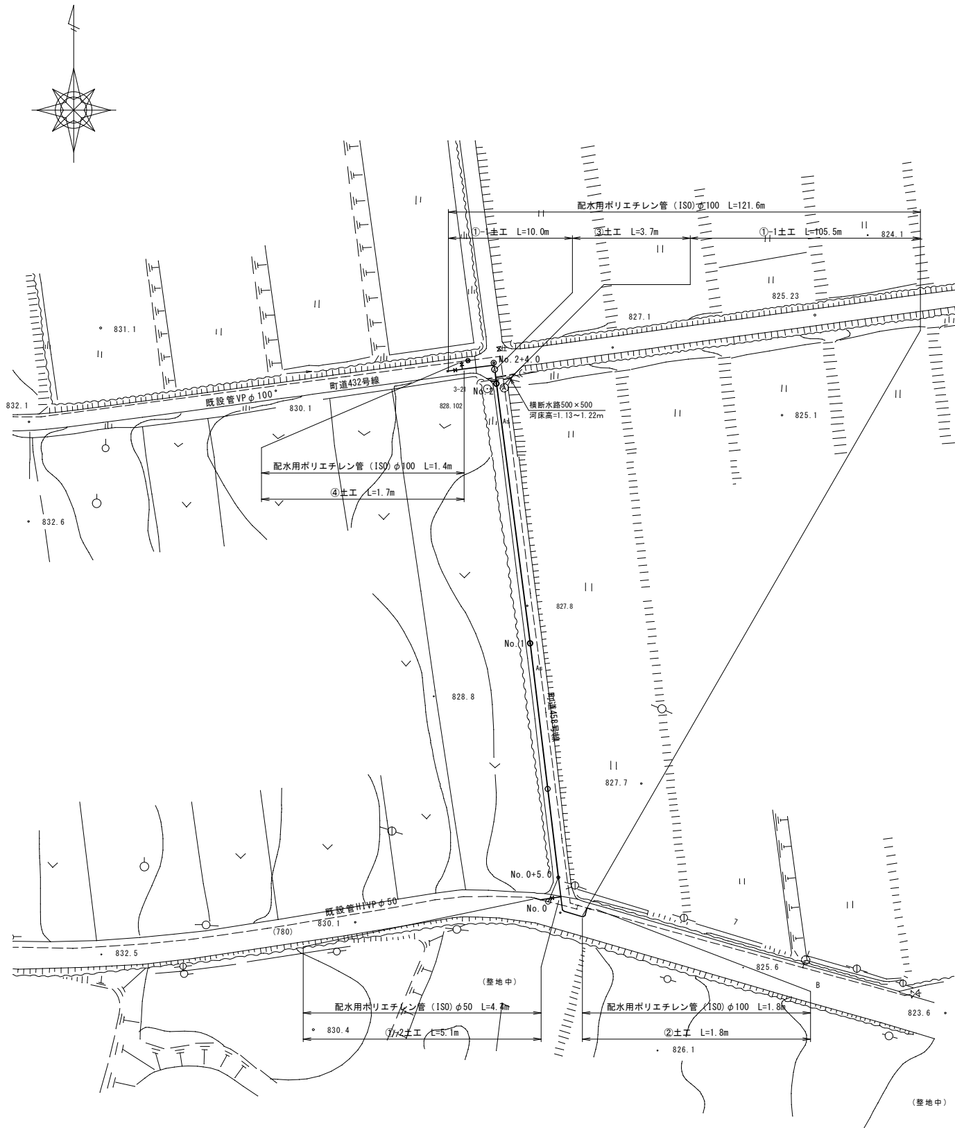
配管平面図 S=1:500
