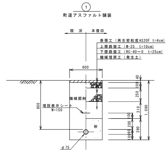
標準掘削断面図 S=1:20
