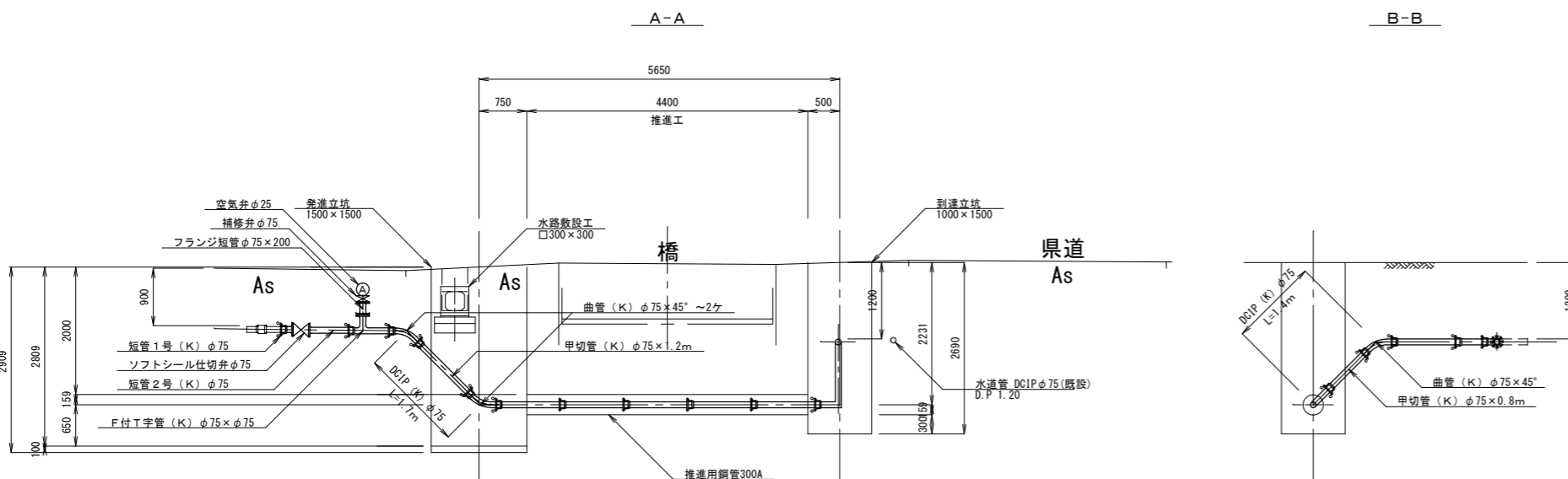
断面図 S=1:50
