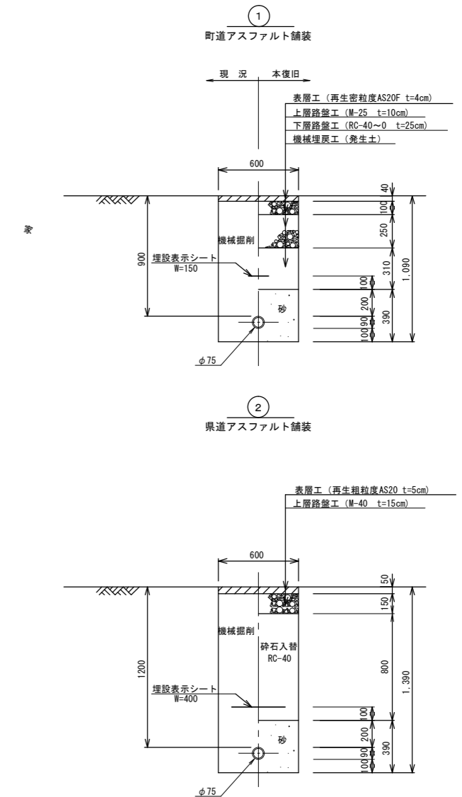
水路敷設標準断面図 S=1:20
