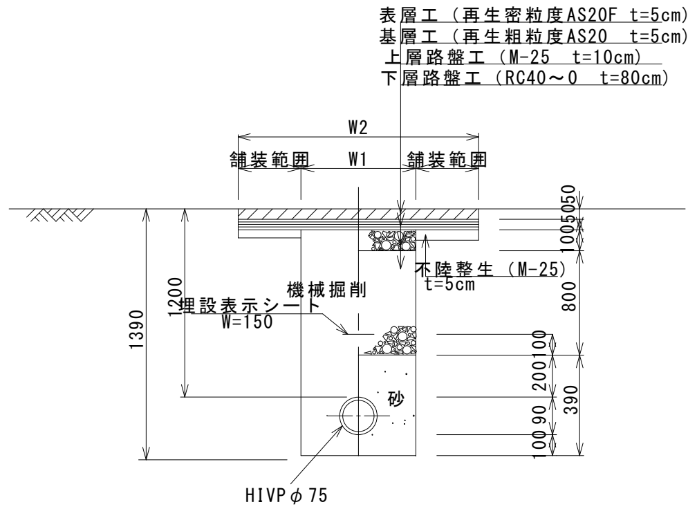
展開図 S = 1/50
