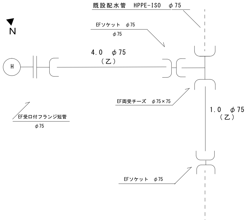
詳細図 S = Free
